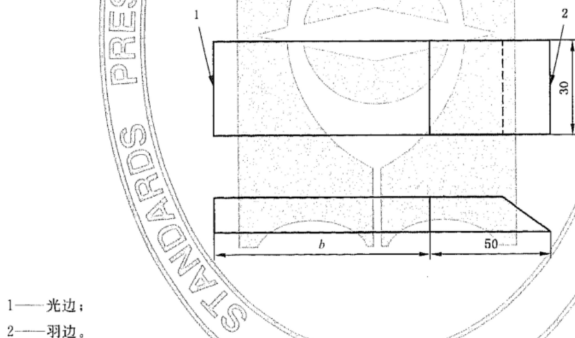
图 B.1 试样切裁示意图
